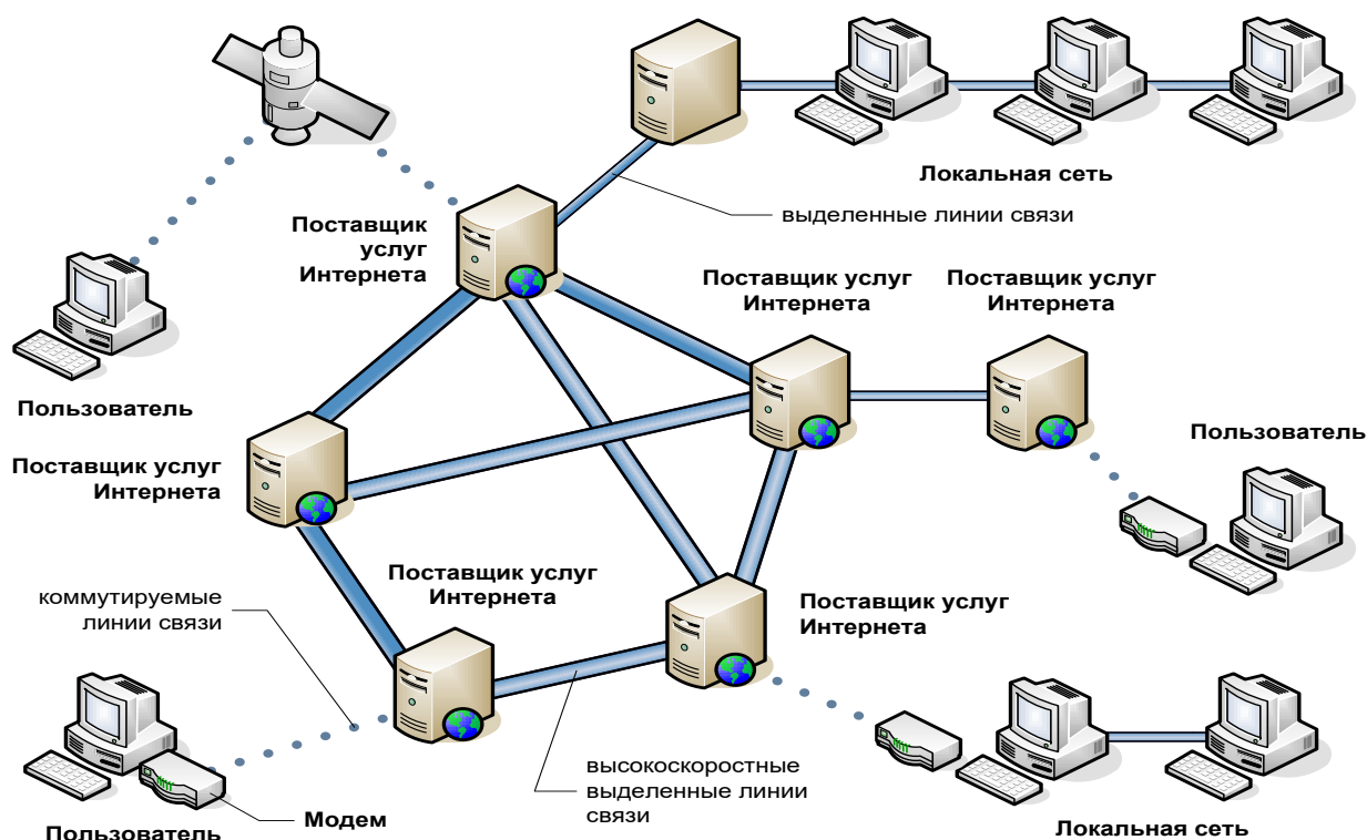
Рис. 1.1. Структура глобальной информационно-телекоммуникационной сети Интернет 2
