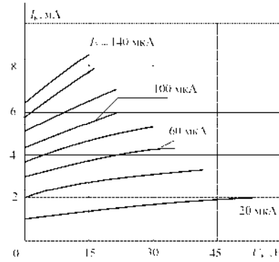
б. Выходные характеристики
