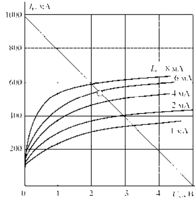
б. Выходные характеристики
