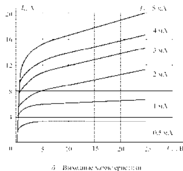
Рис. 12. Характеристики транзистора 2Т 3176 А [3]
