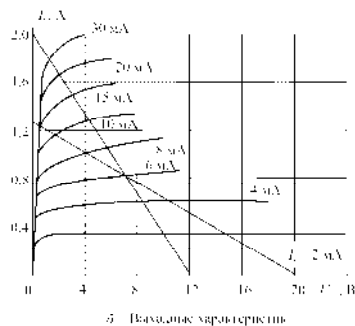
Рис. 11. Характеристики транзистора 2Т 860 А [3]
