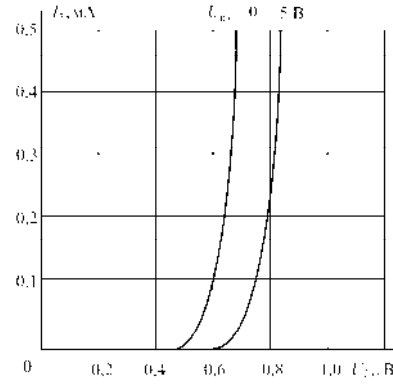
а. Входные характеристики
