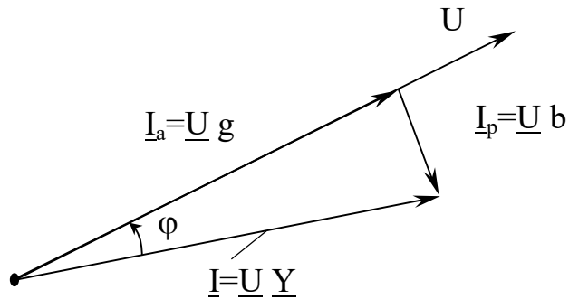
Рисунок 10 – Треугольник тока
