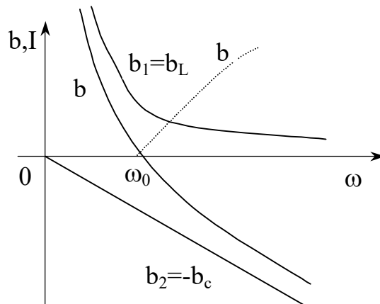
Рисунок 23 – Частотные характеристики параллельного контура.
