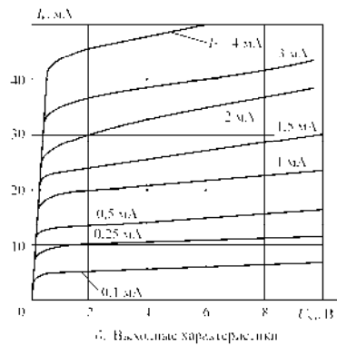
Рис. 11.5 Характеристики транзистора КТ 218 А9
