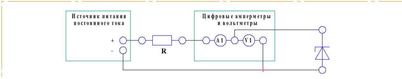
Рисунок 2 – Схема электрических соединений
