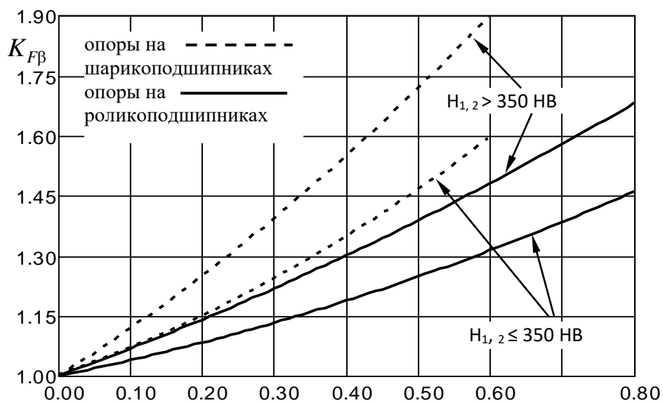
Рис.2.5. Коэффициент концентрации нагрузки для напряжений изгиба (конический одноступенчатый редуктор)
