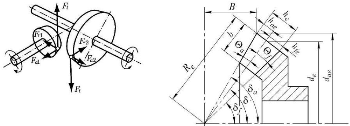
Рис. 2.6. Геометрические параметры конической передачи
