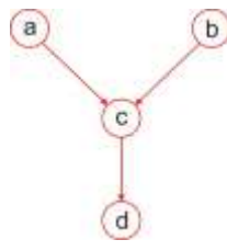
Графическая модель для вероятностной модели 1
