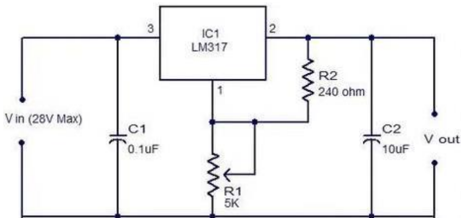
Типовое применение микросхемы в качестве стабилизатора
