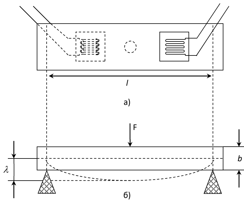
Рис. 3. Схема эксперимента.
