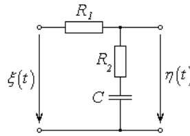
Рисунок 16.1 - Электрическая схема пропорционально-интегрирующего фильтра
