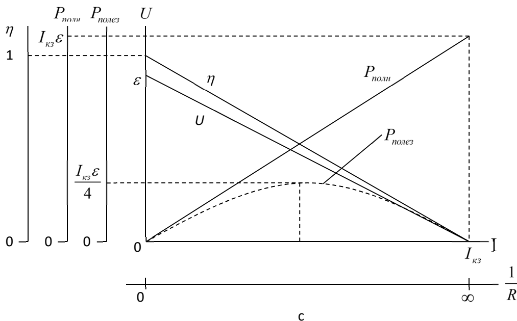
Рис. 1. Зависимость U, P_{\text{полез}}, P_{\text{полн}}, \eta от I \left( \frac{1}{R} \right)
