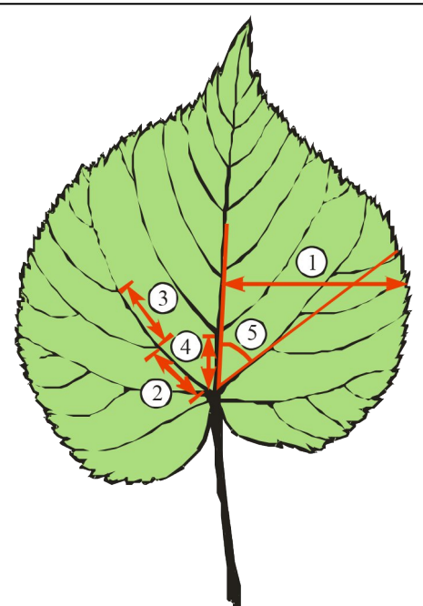
Рис. 3. Схема морфологических признаков, для оценки стабильности развития липы мелколистной ( Tilia cordata )
