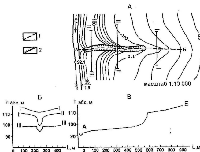
Рис.2. Морфологическое строение оврага в плане (А), его поперечные (Б) и продольный профили (В): 1-1, 11-11, III-III — линии поперечных профилей; А-В — линия продольного профиля; 1 - тальвег; 2 - обрывистые склоны оврага
