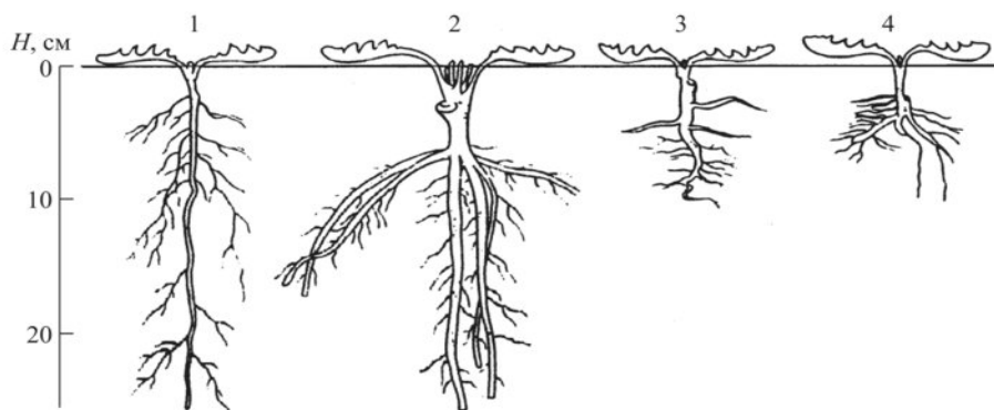
Рисунок 1 - Изменение направления роста корней у одуванчика (Taraxacum) в зависимости от уровня грунтовых вод : 1 – сухой луг; 2 – свежий; 3 – сырой луг; 4 - заболоченная территория
