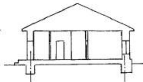
Разрез 0-0 (1:200)
