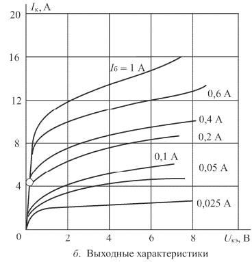
Рис. П1.6 Характеристики транзистора КТ 847 А
