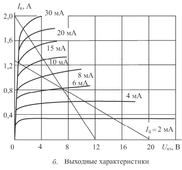
Рис. П.1.1 Характеристики транзистора 2Т 860 (А—В)
