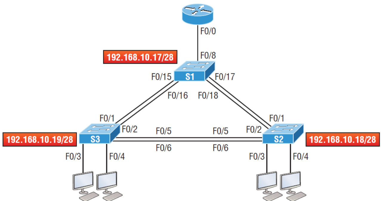
Рисунок 8. Коммутируемая сеть
