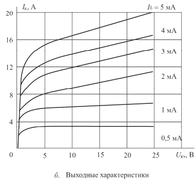
Рис. П.1.2 Характеристики транзистора 2Т 827 (А—В)
