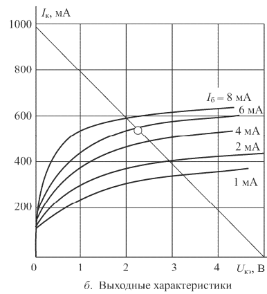
Рис. П.1.3 Характеристики транзистора КТ 3176 А9
