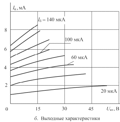
Рис. П.1.4 Характеристики транзистора КТ 216 А
