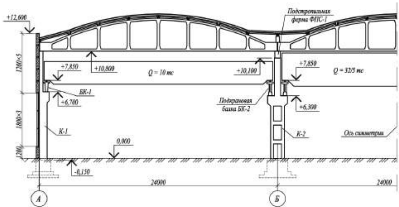
Поперечный разрез здания
