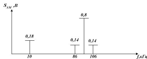
Рисунок 5— Спектральная диаграмма
