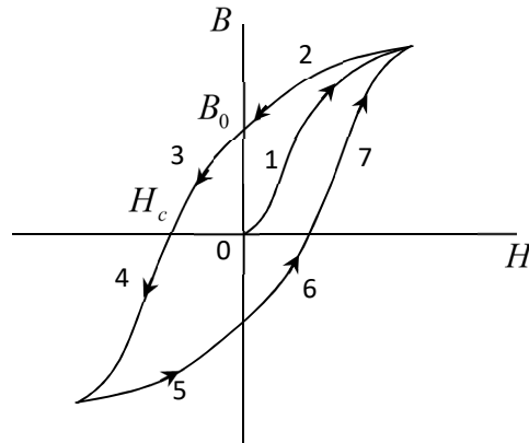
Рис. 2. Кривая гистерезиса
