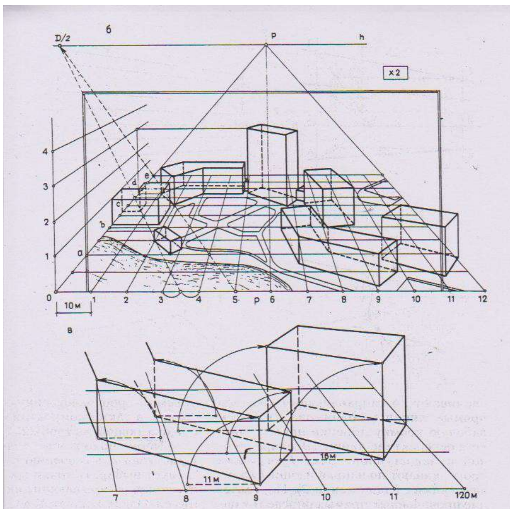
Задание 14. Графическая работа «Перспектива геометрических тел, перспектива моделей»
