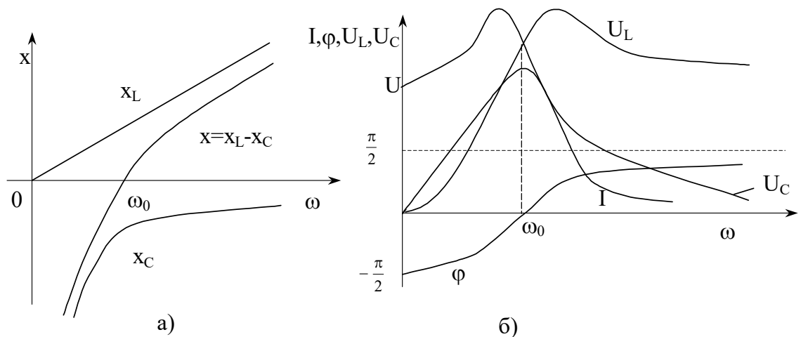
Рисунок 19 – Частотные и резонансные характеристики последовательной цепи
