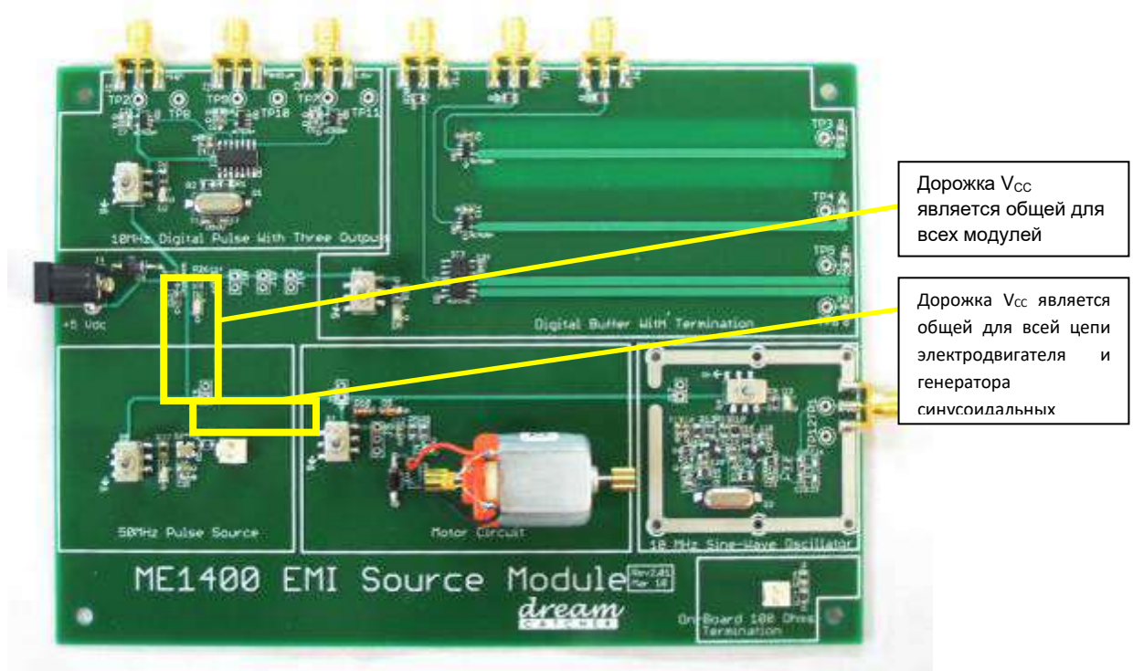
Рисунок 8. Компонировка дорожки V_{CC}
