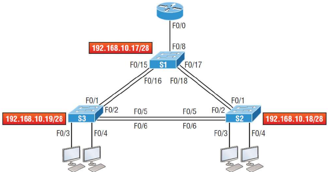
Рисунок 8. Коммутируемая сеть
