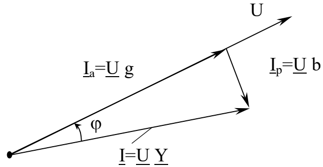
Рисунок 10 – Треугольник тока
