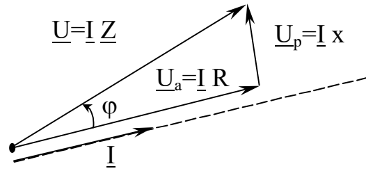
Рисунок 8 – Треугольник напряжений
