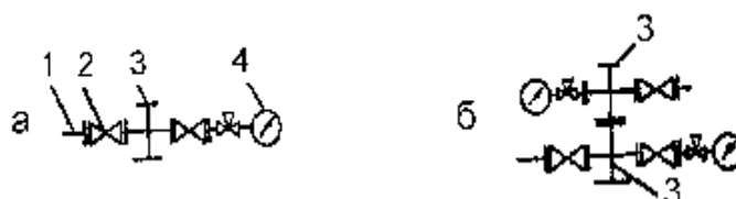
Рис. 3.2. Схемы трубных обвязок фонтанной арматуры:
