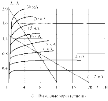
Рис. 11.1. Характеристики транзистора 2Т 8601 А — 3И
