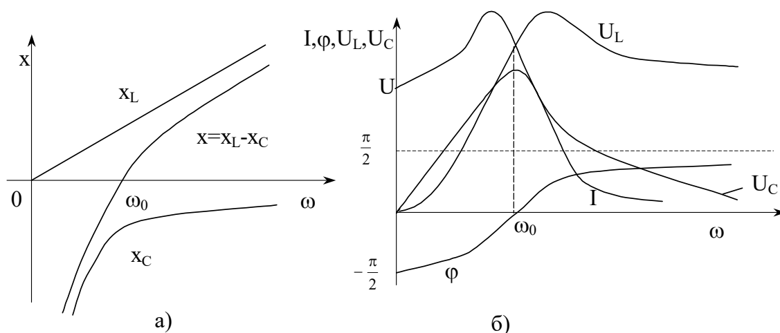
Рисунок 19 – Частотные и резонансные характеристики последовательной цепи
