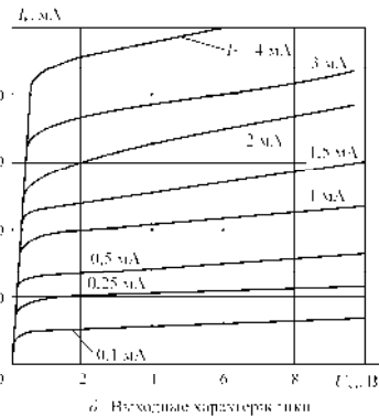
Рис. 11.5 Характеристики транзистора КТ 218А9 — 191
