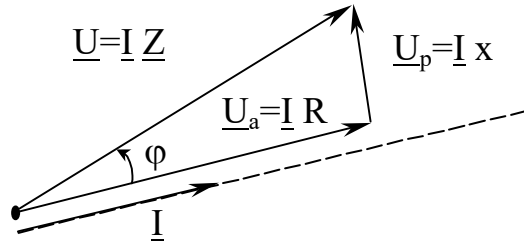
Рисунок 8 – Треугольник напряжений
