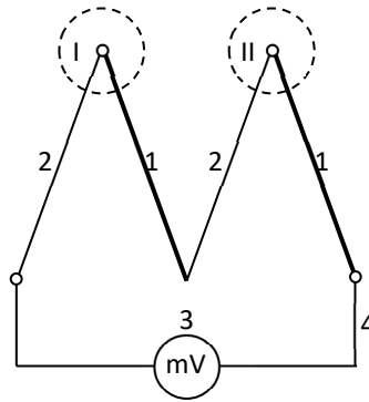
Рис. 2. Измерительная схема цепи термопары. I – область измеряемой температуры, II – термостатированная область,
