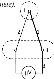
Рис. 3. Измерительная схема цепи термопары (2). I – область измеряемой температуры; II – область температуры лаборатории.
