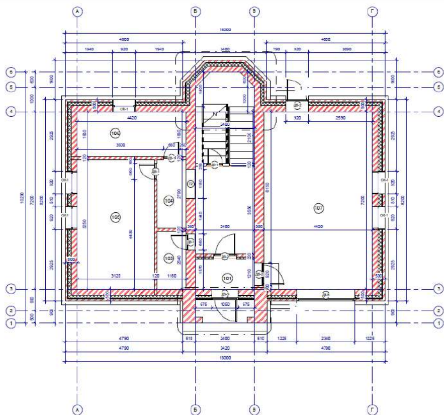
план 1 этажа
