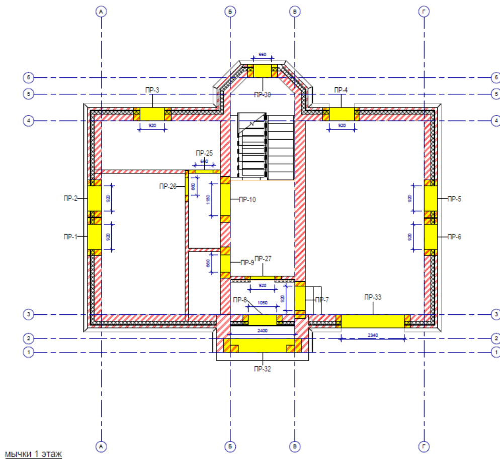
МЫШКИ 1 ЭТАЖ
