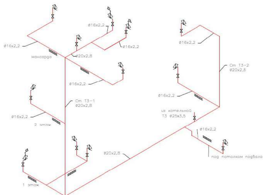
схема ТЗ
