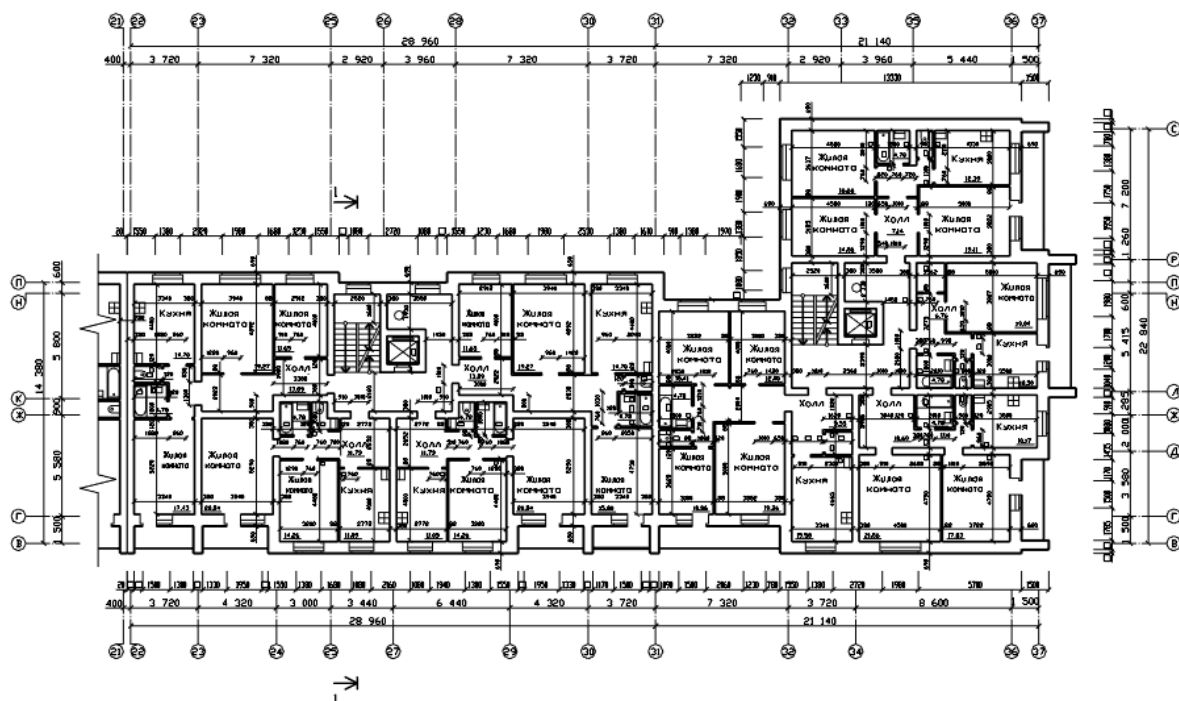
ПЛАН ТИПОВОГО ЭТАЖА В ОСЯХ 22-37
