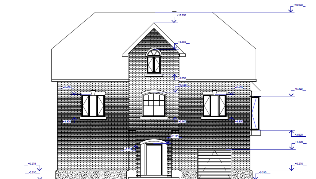
фасад А-Г
