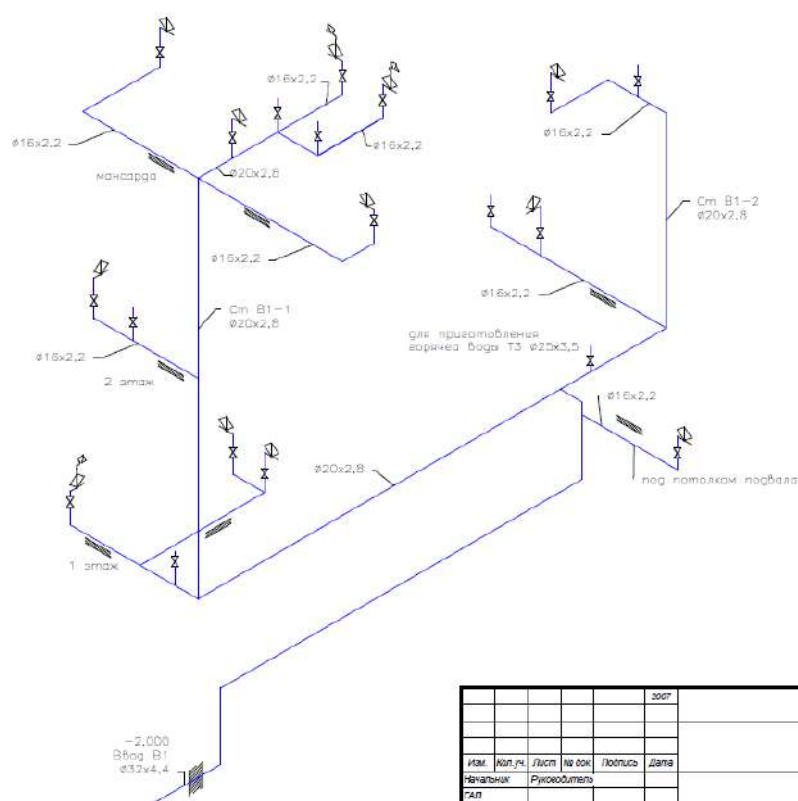
схема В1
