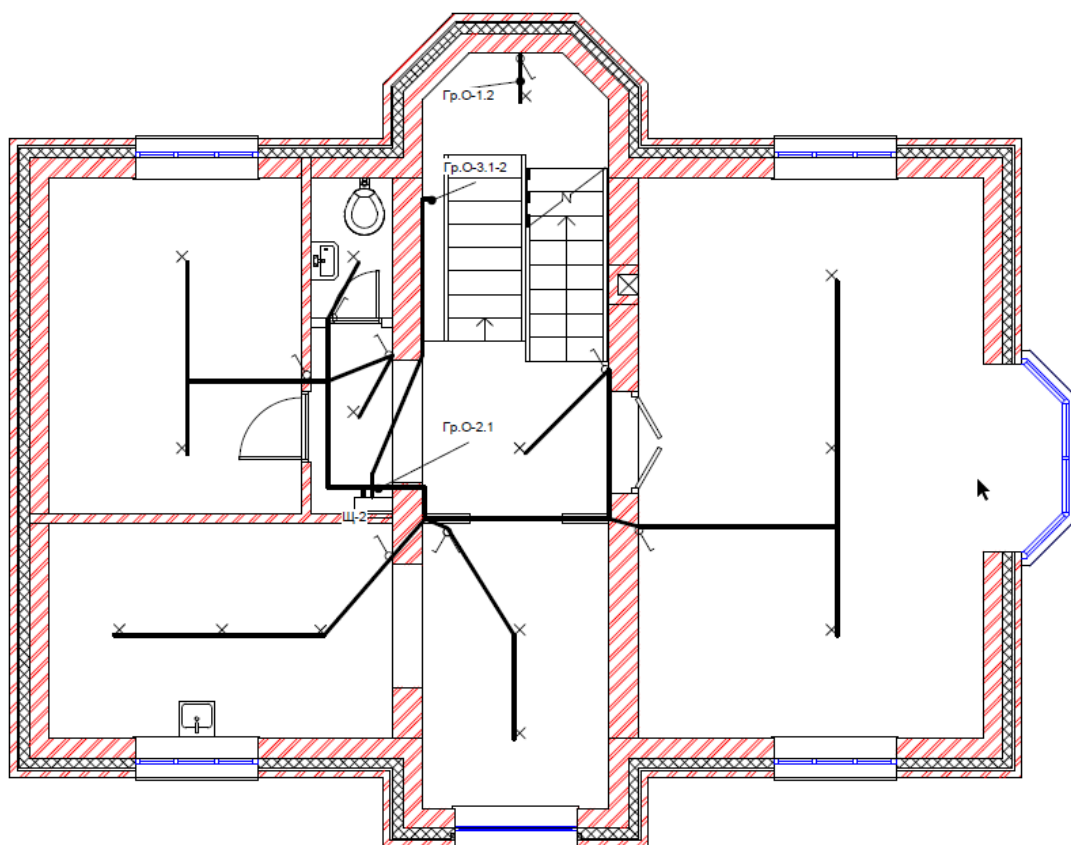
2 этаж - освещение
